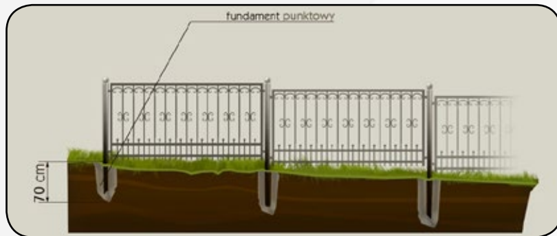
Montage bei einem Geländegefälle.
