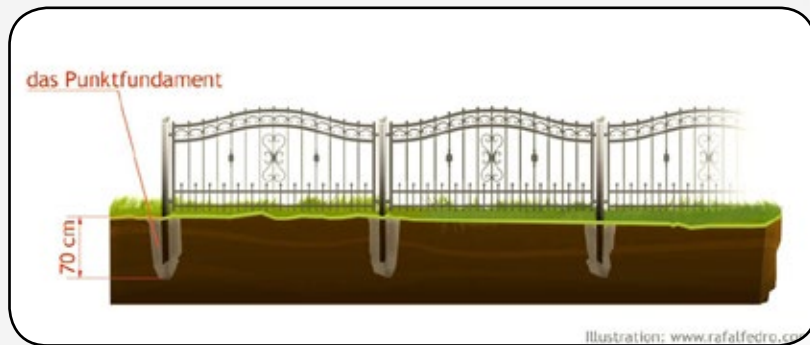
Zaun montiert in die Erde in gerader Linie.
